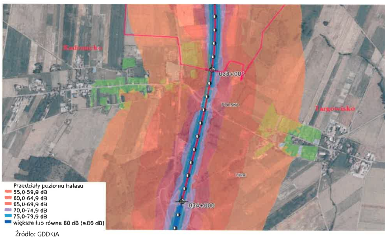
Rysunek 4 Mapa hałasu wzdłuż drogi S5 dla miejscowości Radomicko oraz Targowisko
