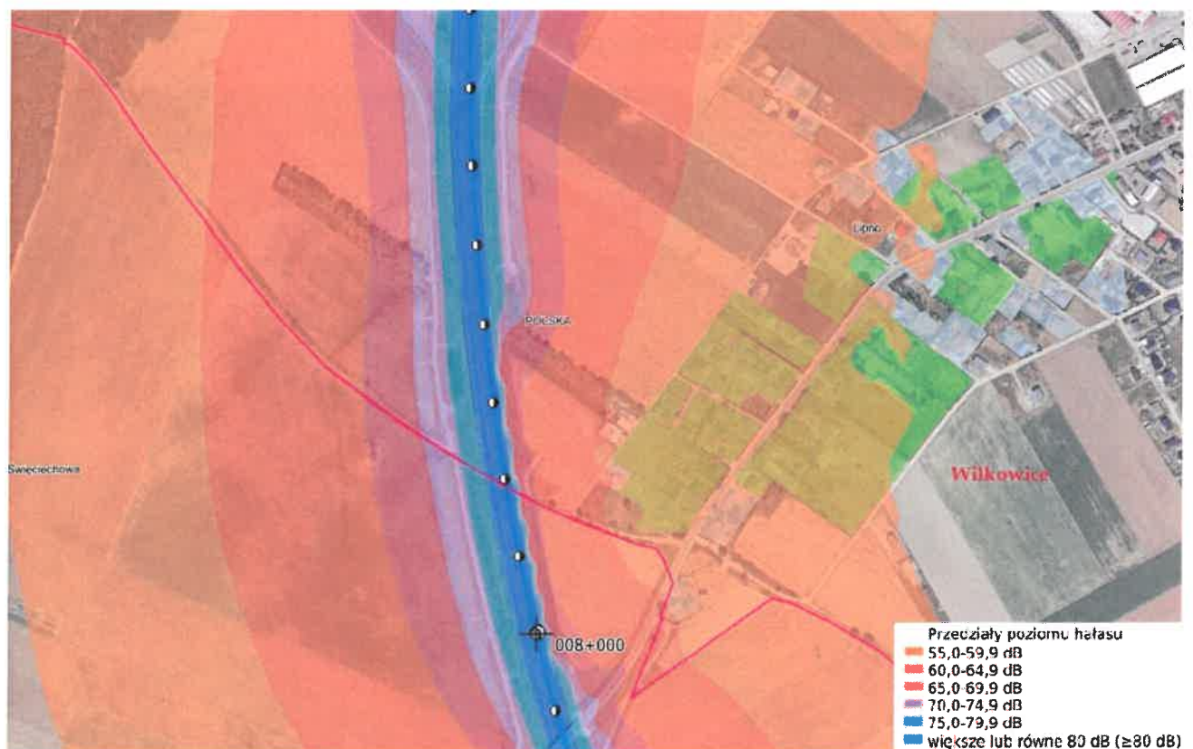
Rysunek 7 Mapa hałasu wzdłuż drogi S5 dla miejscowości Wilkowice
