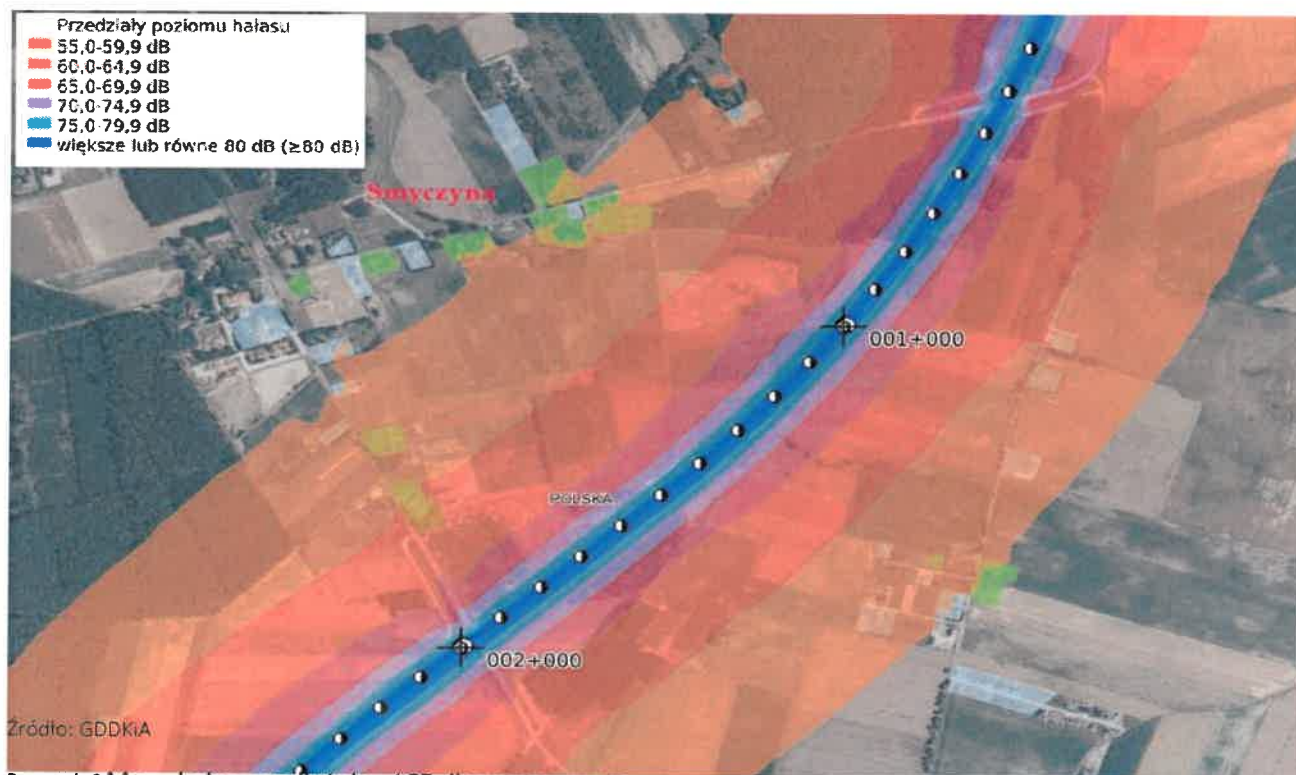
Rysunek 6 Mapa hałasu wzdłuż drogi S5 dla miejscowości Mórkowo
