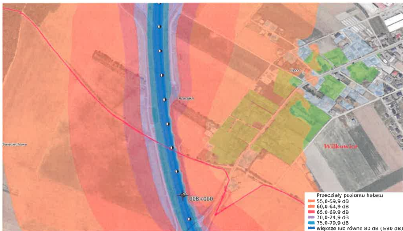
Rysunek 7 Mapa hałasu wzdłuż drogi S5 dla miejscowości Wilkowice
