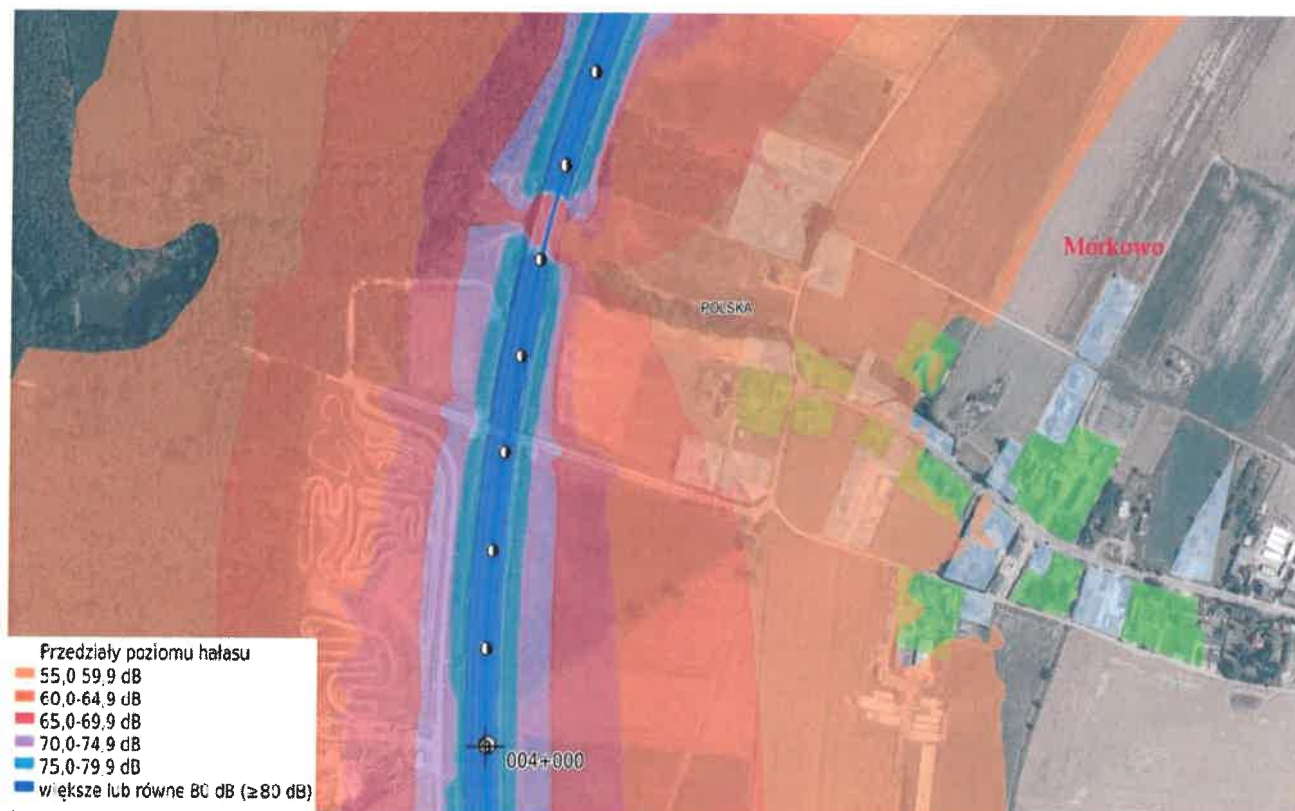
Rysunek 6 Mapa hałasu wzdłuż drogi S5 dla miejscowości Morkowo
