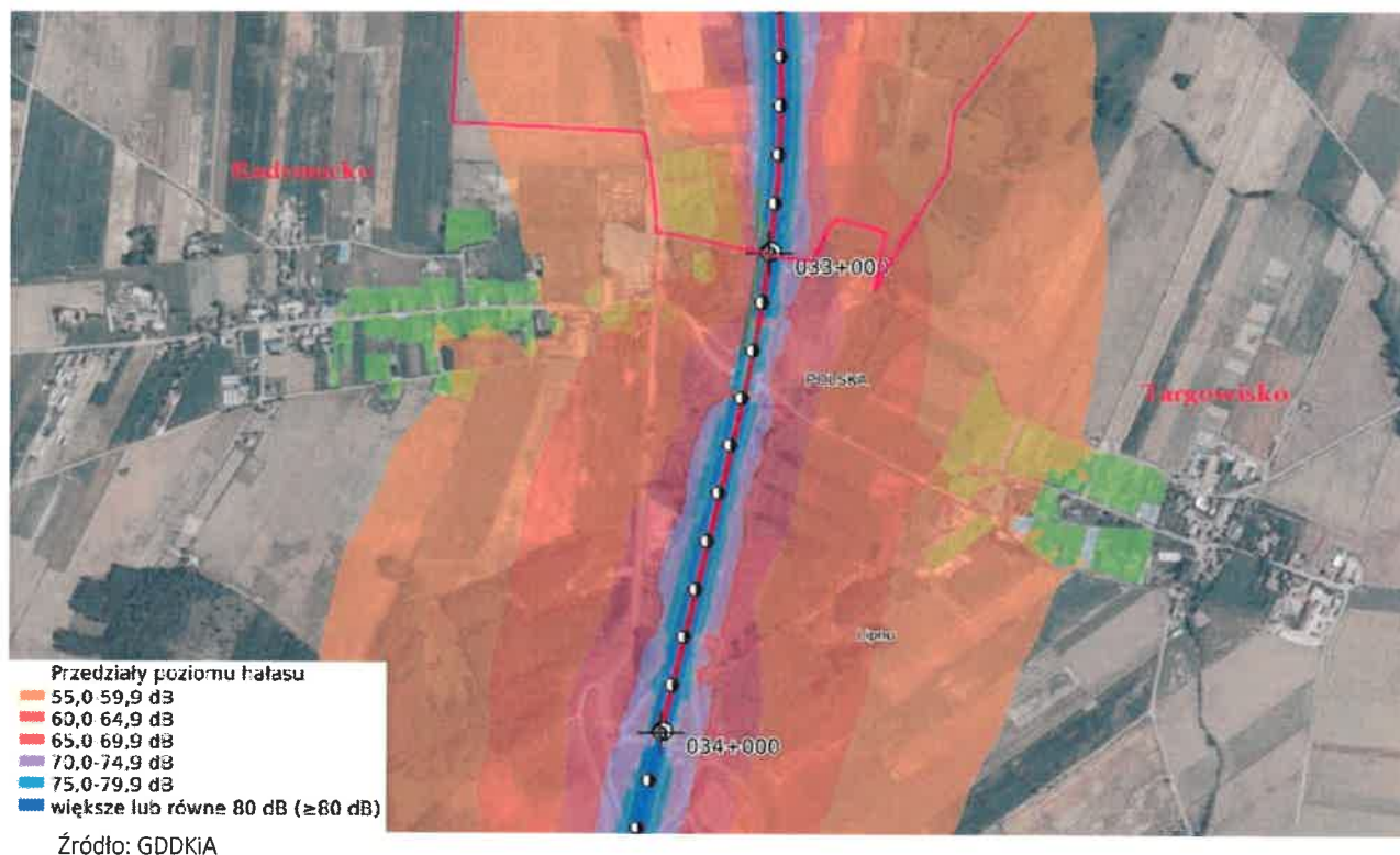
Rysunek 5 Mapa hałasu wzdłuż drogi S5 dla miejscowości Smyczyna
